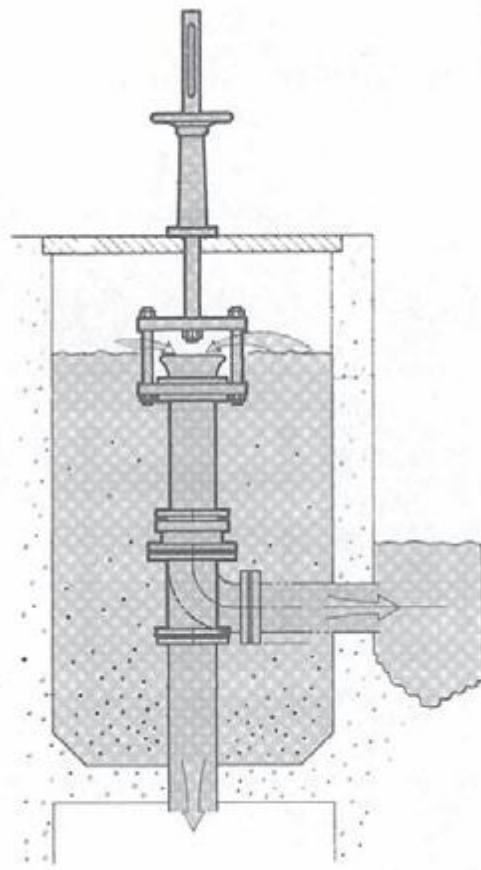
Fig46 テレスコープ弁
