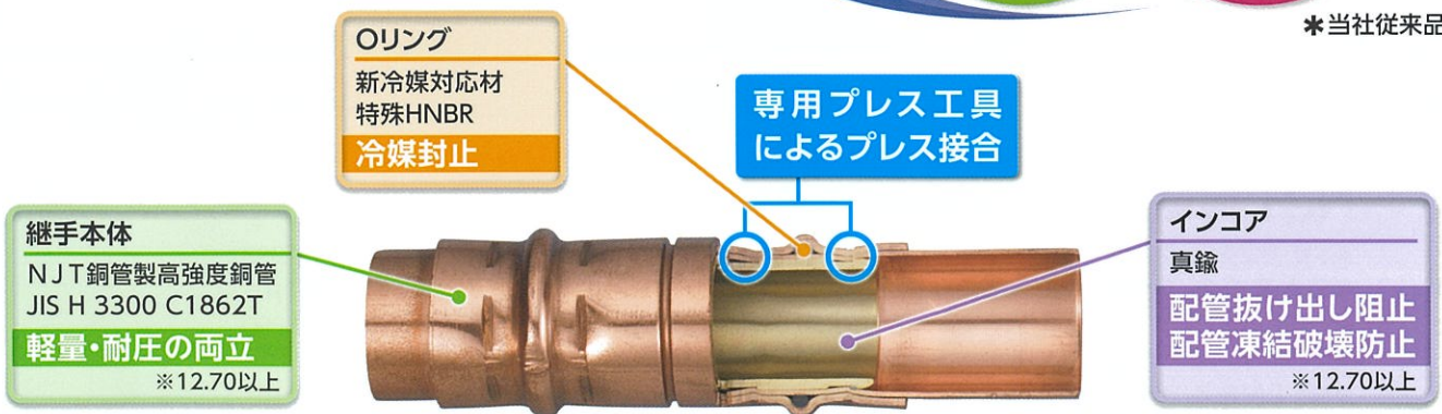
RGプラスの構造
